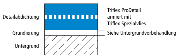
Systemaufbau – Detail A
